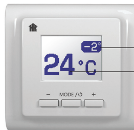
Рис. 4 Индикация в режиме корректировки показаний датчика температуры воздуха
